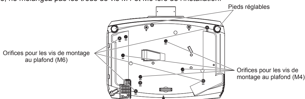
Positions des orifices pour les vis de montage au plafond et des pieds réglables
